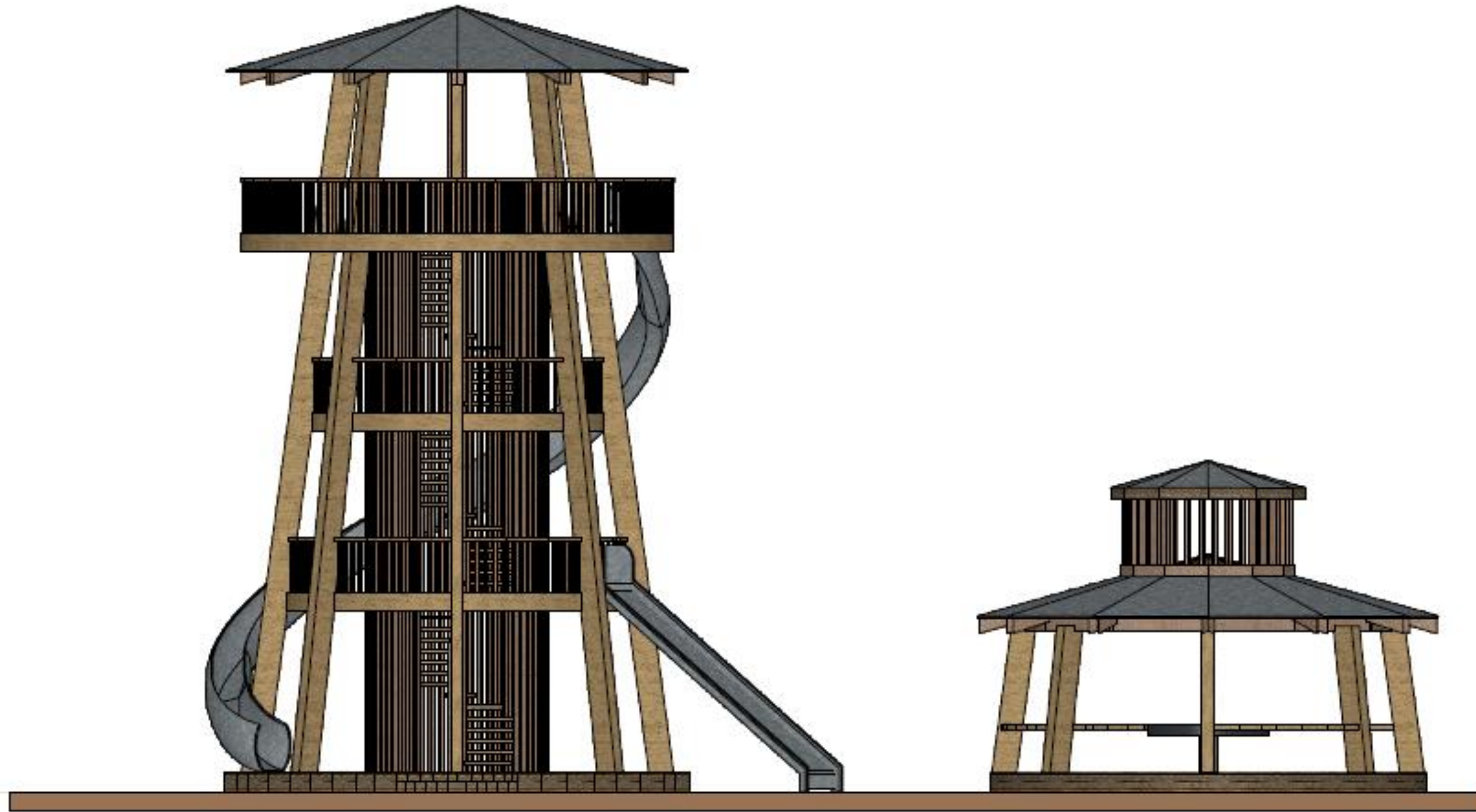
Ansicht Süd
